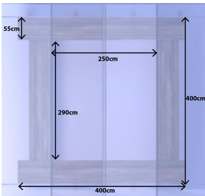
Afbeelding 3: 1 standplaats food – bovenaanzicht (2 markkramen tegen elkaar aan, met planken rondom gelegd)
