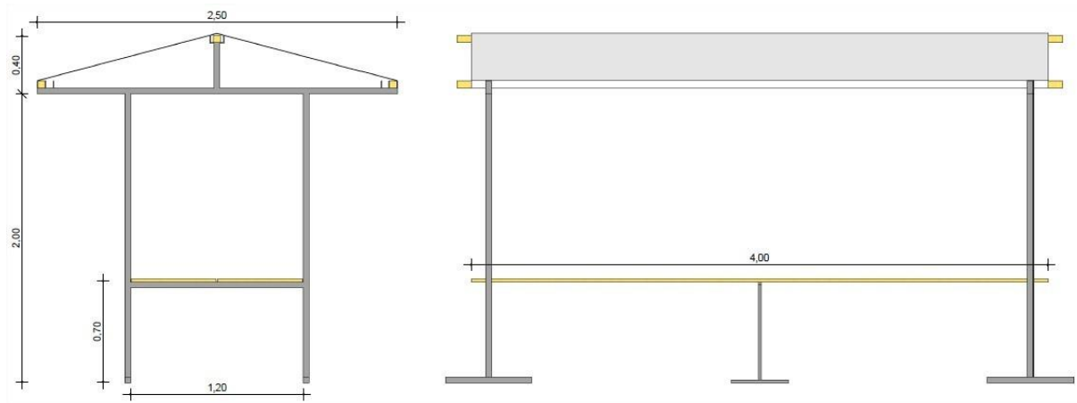
Afbeelding 1: non-food kraam voor- en zijaanzicht
