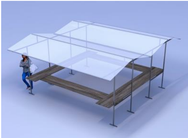
Afbeelding 2: 1 standplaats food - 3D aanzicht (2 markkramen tegen elkaar aan, met planken rondom gelegd)
